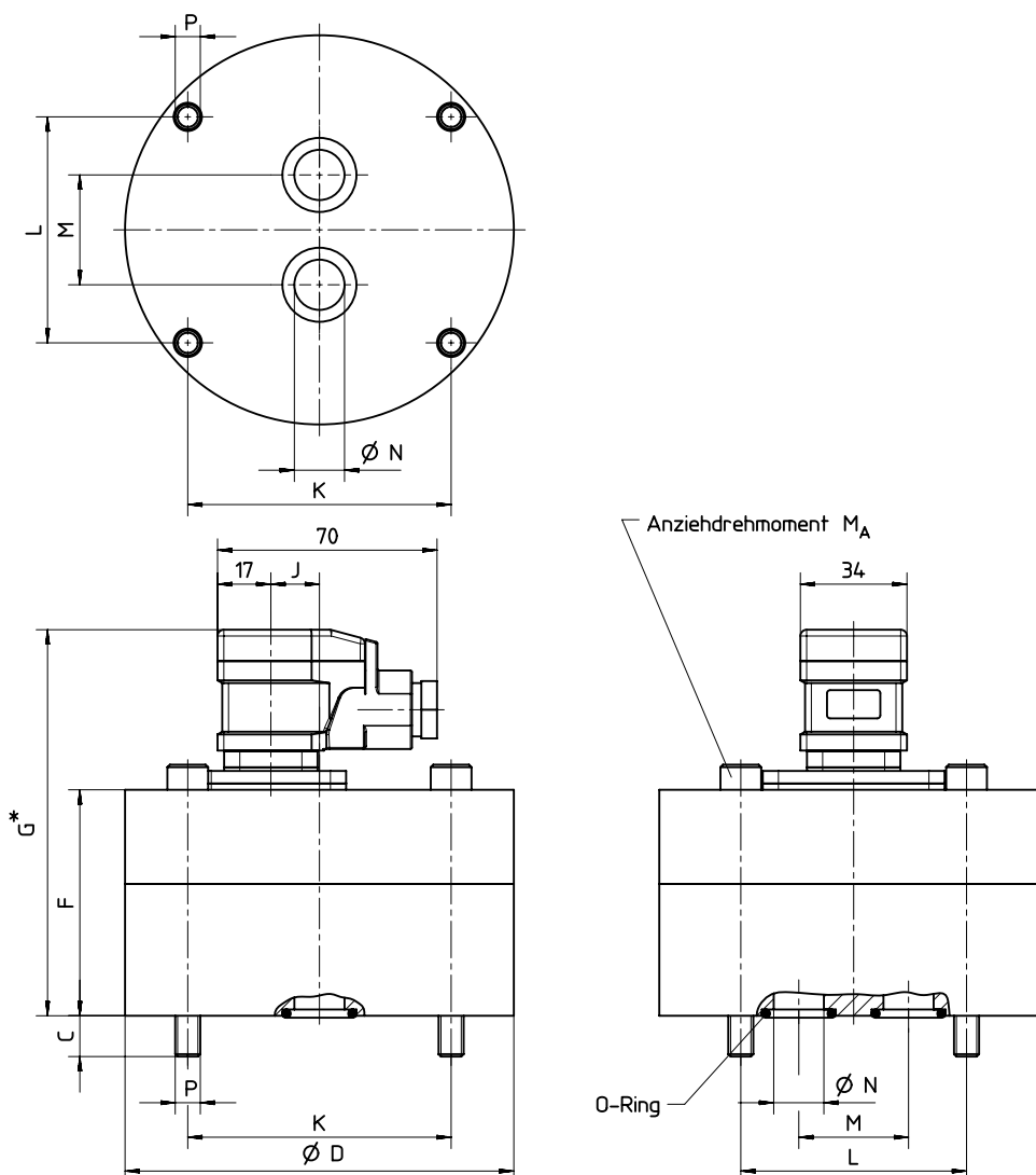
Anschlussmaße
