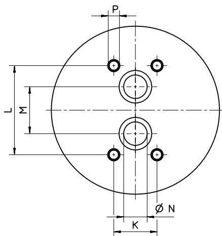
Anschlussmaße
