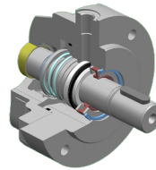
Gleitringdichtung mit Radialwellendichtring und Anschlussbohrung für Flüssigkeitsvorlage
