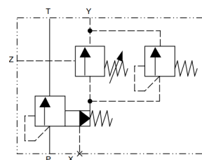
Schaltsymbol ausführlich
