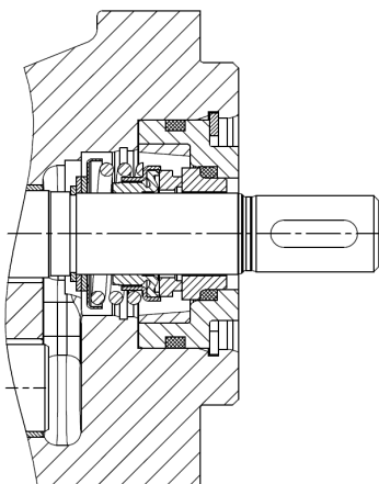
Gleitringdichtung Dichtungsart: 34; 35; 40
