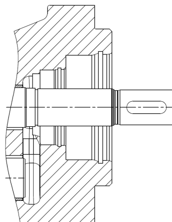
ohne Wellenabdichtung (Leckölabführung durch Wellenabdichtungsraum) Dichtungsart: 30; 36
