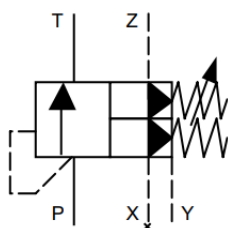
Schaltsymbol vereinfacht
