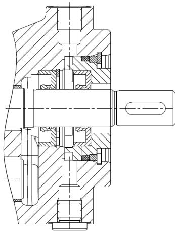
Doppel-Radialwellendichtring Anschlussbohrung G 1/8 (für Flüssigkeitsvorlage) Dichtungsart: 7
