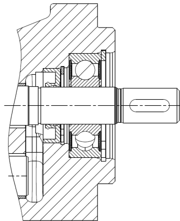
Radialwellendichtring mit Wälzlager Dichtungsart: 1; 2
