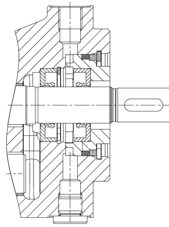
Doppel-Radialwellendichtring (für Vakuumbetrieb) Anschlussbohrung G 1/8 (für Flüssigkeitsvorlage) Dichtungsart: 7; Sondernummer: 74
