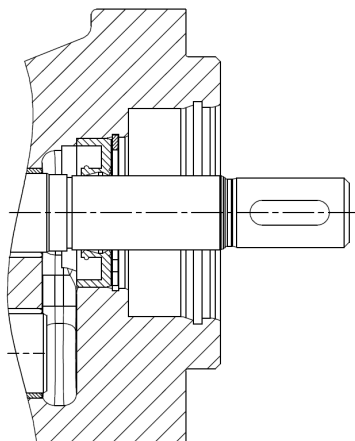
Radialwellendichtring Dichtungsart: 1; 2
