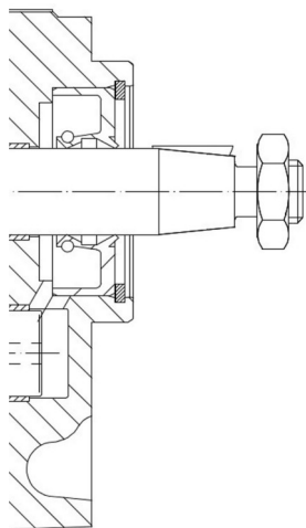
Bague d'étanchéité radiale Types de joints d'étanchéité: 1; 2
