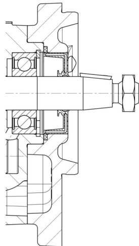
Bague d'étanchéité radiale avec pa- lier aditionnel, modèle léger Types de joints d'étanchéité: 1; 2
