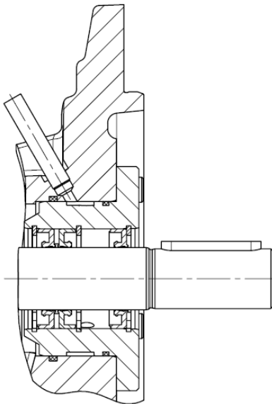
三重径向轴密封圈
