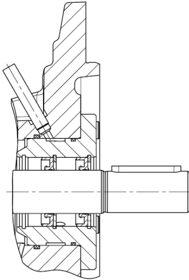
双径向轴密封圈
