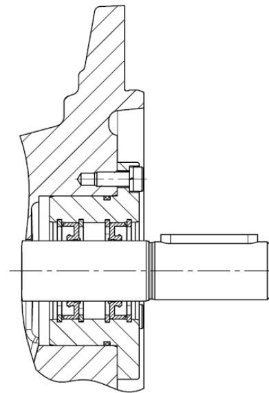
双径向轴密封圈
