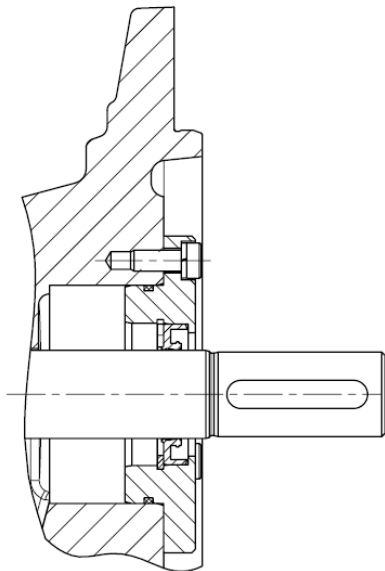
径向轴密封圈 (用于 真空运行)
