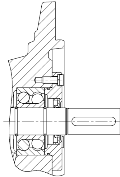
径向轴密封圈 带 滚动轴承
