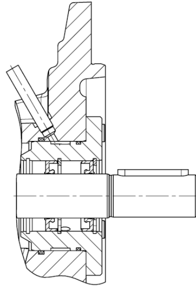
双径向轴密封圈 (用于 真空运行)
