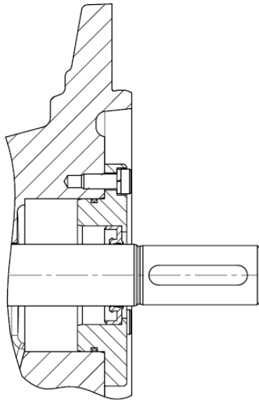
径向轴密封圈
